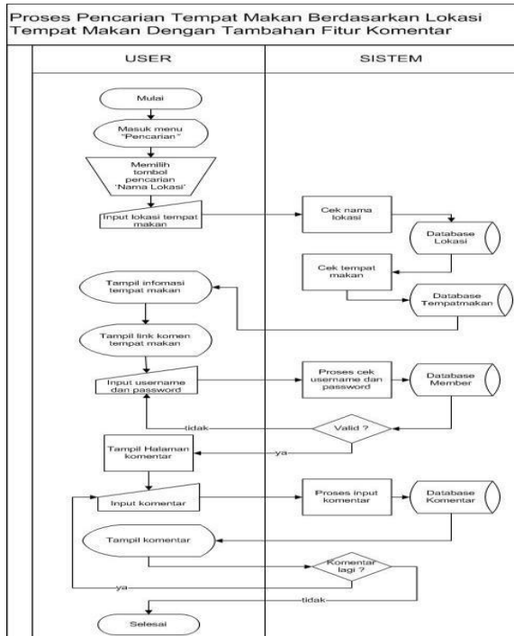
Gambar 2 Flowmap Proses Pencarian Tempat Makan Berdasarkan Lokasi Tempat Makan Dengan Tambahan Fitur Komentar
