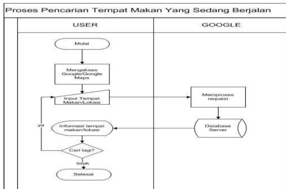
Gambar 1 Proses Pencarian Tempat Makan Yang Sedang Berjalan
