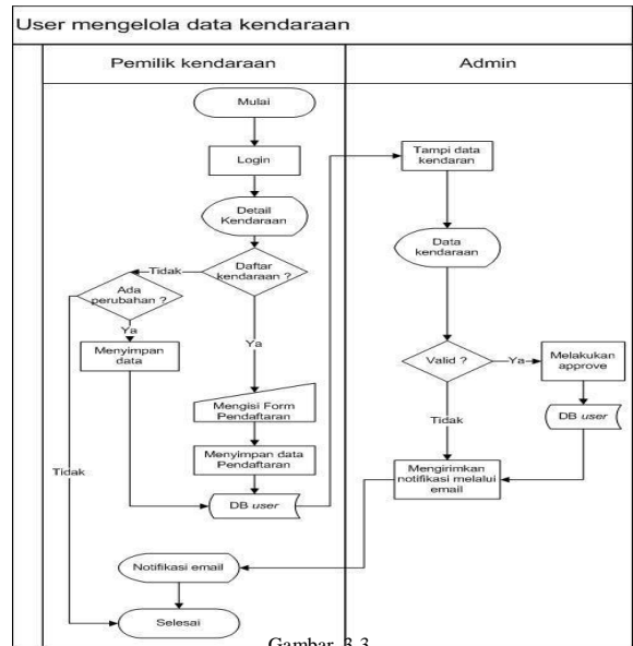
Gambar 3-3 User mengelola kendaraan
