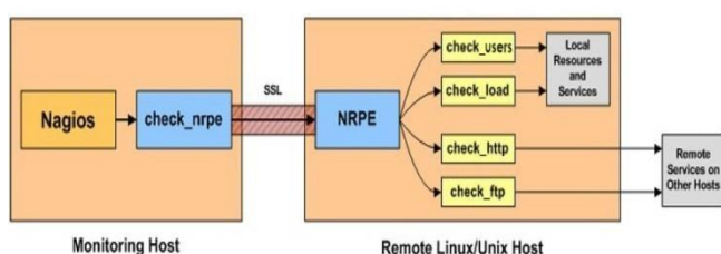
Gambar 3. 3 Cara Kerja Nagios [10]
