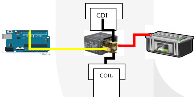
Gambar 3.7 Perancangan relay
