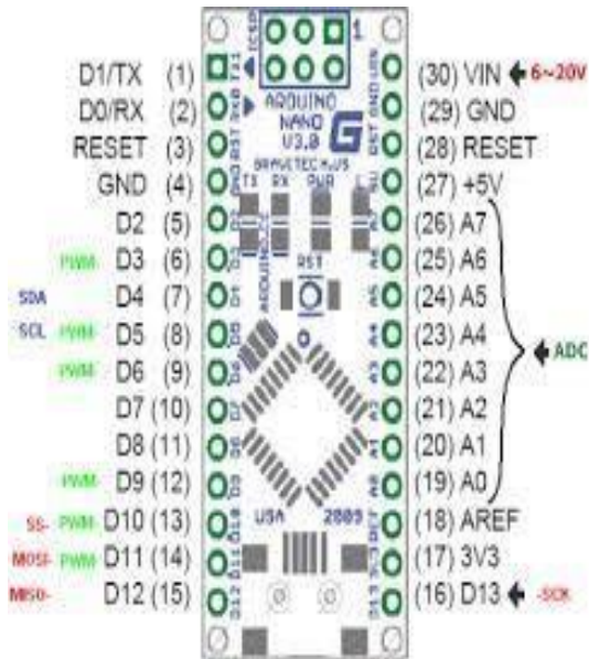
Gambar 2 Arduino Nano v3
