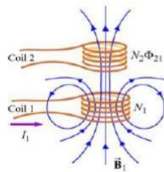
Gambar 2.61 Induksi Bersama
