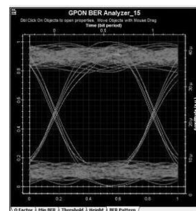
Gambar 5 Eye Diagram GPON link upstream pada titik terjauh
