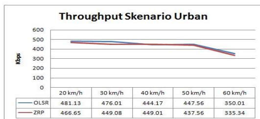
Gambar 4.8 Pengaruh kecepatan node untuk Throughput pada skenario URBAN
