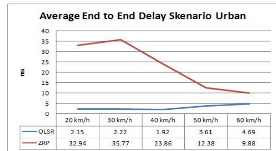
Gambar 4. 6 Pengaruh kecepatan node untuk Delay pada skenario URBAN
