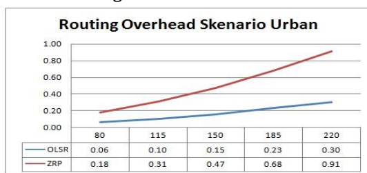
Gambar 4.12 Pengaruh jumlah node terhadap R.O di skenario URBAN
