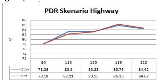
Gambar 4.9 Pengaruh jumlah node terhadap PDR pada skenario Highway
