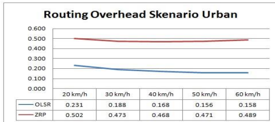
Gambar 4. 4 Pengaruh kecepatan node untuk RO pada skenario URBAN
