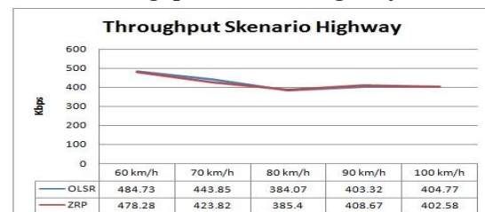
Gambar 4. 7 Pengaruh kecepatan node untuk Throughput pada skenario HIGHWAY
