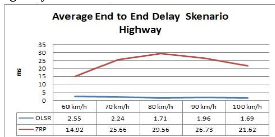
Gambar 4. 5 Pengaruh kecepatan node untuk Delay pada skenario HIGHWAY
