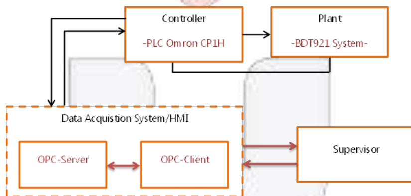
Gambar 1. Sistem SCADA yang Dibangun
