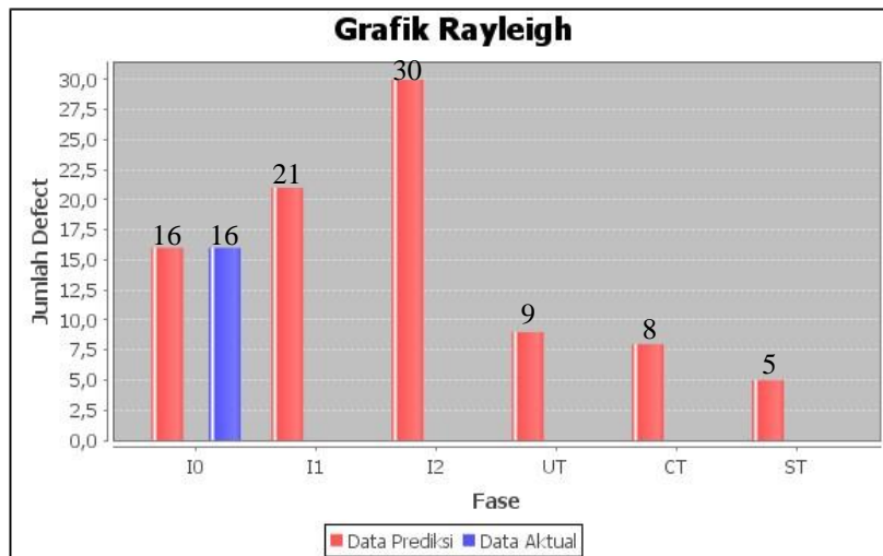
Gambar 3. Grafik prediksi aplikasi web Prosys
