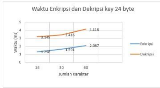
Gambar 4.3 Perbandingan Waktu Enkripsi dan Dekripsi Key 24 Byte
