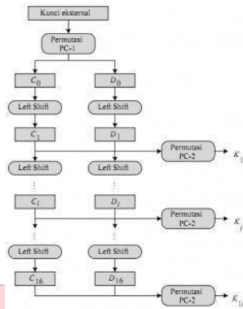
Gambar 2.2 Skema Pembangkitan Kunci Internal Algoritma DES [3]
