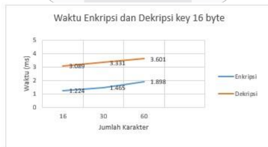
Gambar 4.2 Perbandingan Waktu Enkripsi dan Dekripsi Key 16 Byte
