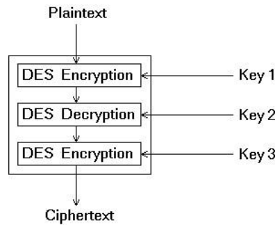
Gambar 2.4 Prosedure enkripsi pada triple DES [5]
