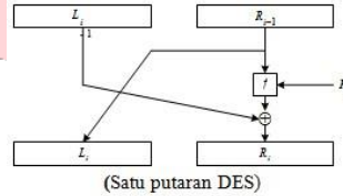
Gambar 2.3 Skema 1 putaran DES [3]
