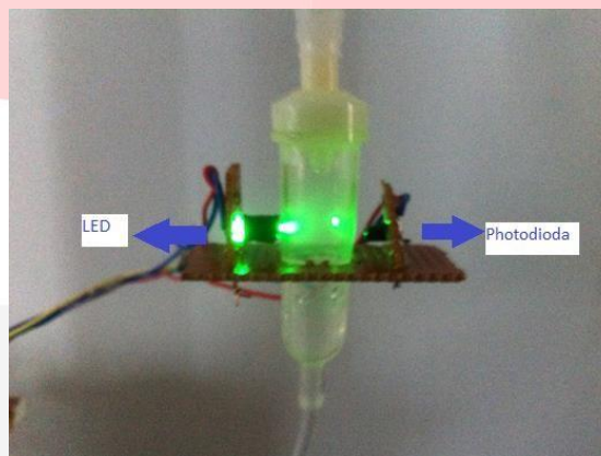
Gambar 3.3 Sensor photodiode pada tabung infus
