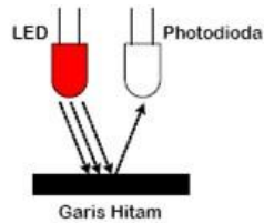
Gambar 1. Cahaya pantulan sedikit
