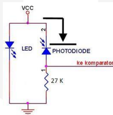
Gambar 3.1 Sensor Photodiode tidak terkena cahaya
