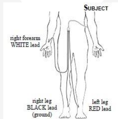
Gambar 4.2 Titik Sadapan data untuk EKG
