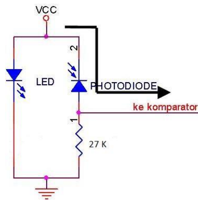
Gambar 3.2 Sensor Photodiode terkena cahaya
