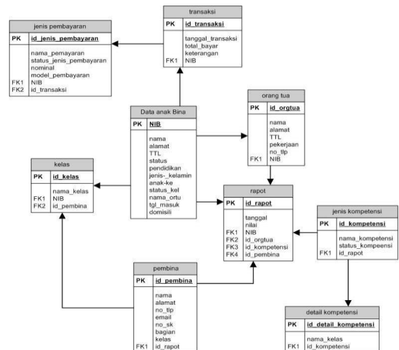
Gambar 5 Skema Relasi
