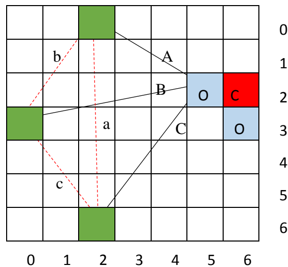
Gambar 3.3 Penghitungan F-Cost
