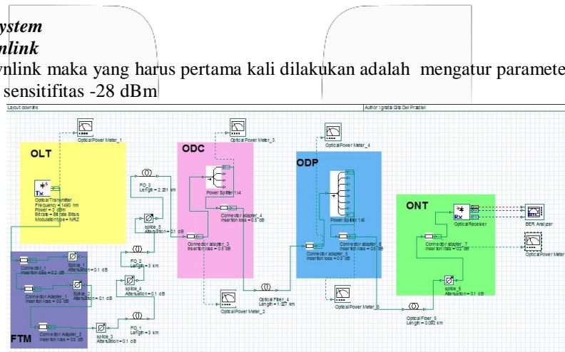
Gambar 4.1 Konfigurasi Downlink
