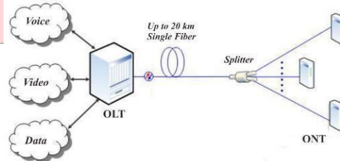
Gambar 2.1 Arsitektur GPON
