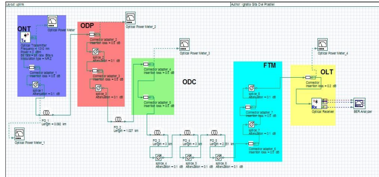
Gambar 4.2 Konfigurasi Uplink
