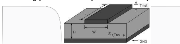
Gambar 2.2 Teknik Pencatutan Microstrip Line
