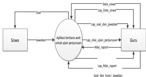
Gambar 2 Diagram Konteks
