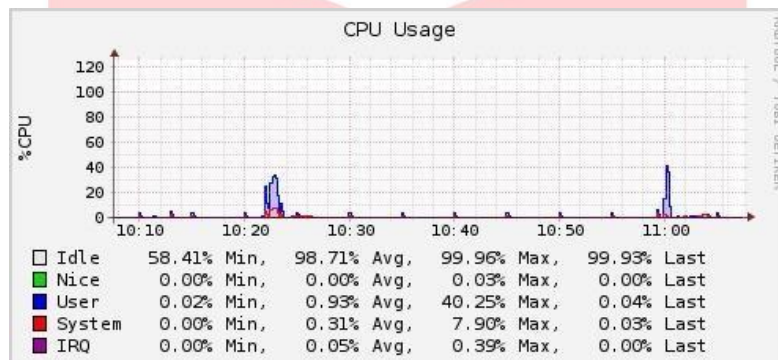
Gambar 3. Grafik persentase penggunaan CPU
