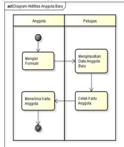
Gambar 3.16 Diagram Aktivitas Anggota Baru
