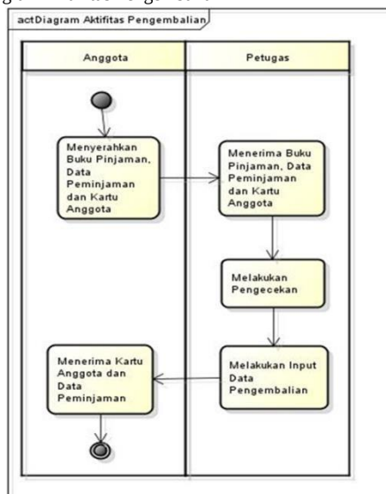
Gambar 3.15 Diagram Aktivitas Pengembalian
