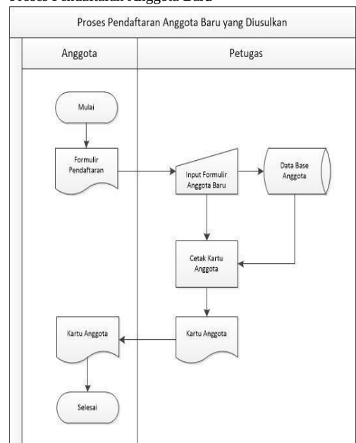
Gambar 3.7 Flowmap Pendaftaran Anggota Baru yang Diusulkan
