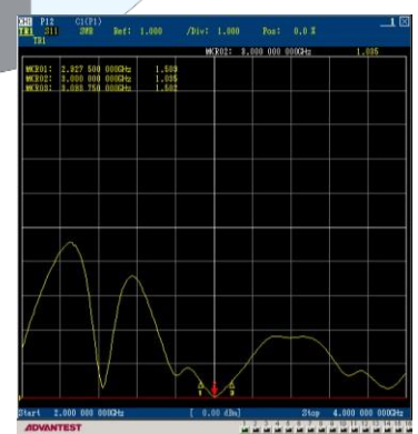
Gambar 10. Grafik VSWR
