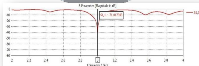
Gambar 6. Grafik return loss
