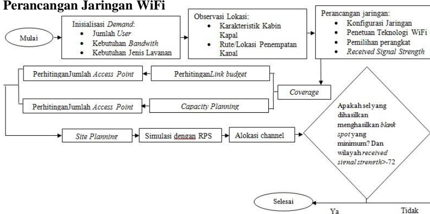
Gambar 1. Diagram Alir Perancangan Jaringan WiFi
