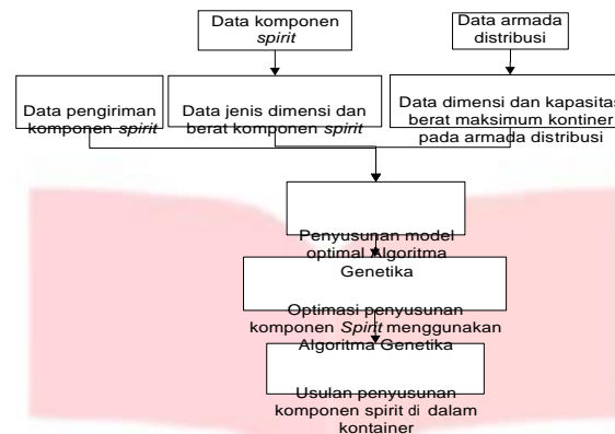
Gambar III.1 Identifikasi Masalah
