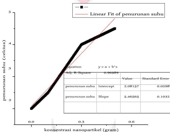
Gambar 3.4 Grafik penurunan suhu terhadap konsentrasi nanopartikel.
