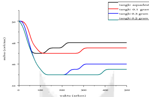
Gambar 3.3 (a) Grafik penurunan suhu pada tangki.
