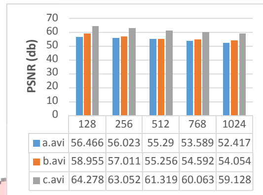
Gambar 9. Hasil Pengujian PSNR
