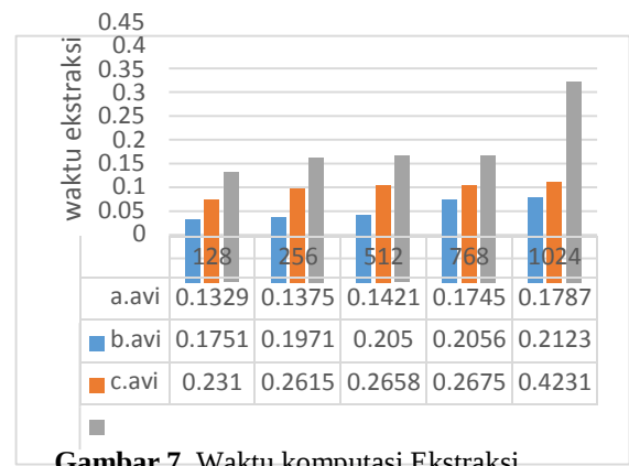
Gambar 7. Waktu komputasi Ekstraksi
