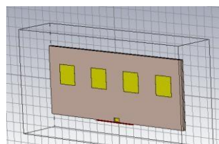
Gambar 3. 1 Simulasi Antena susunan 4 elemen proximity coupled dengan teknik matching impedance
