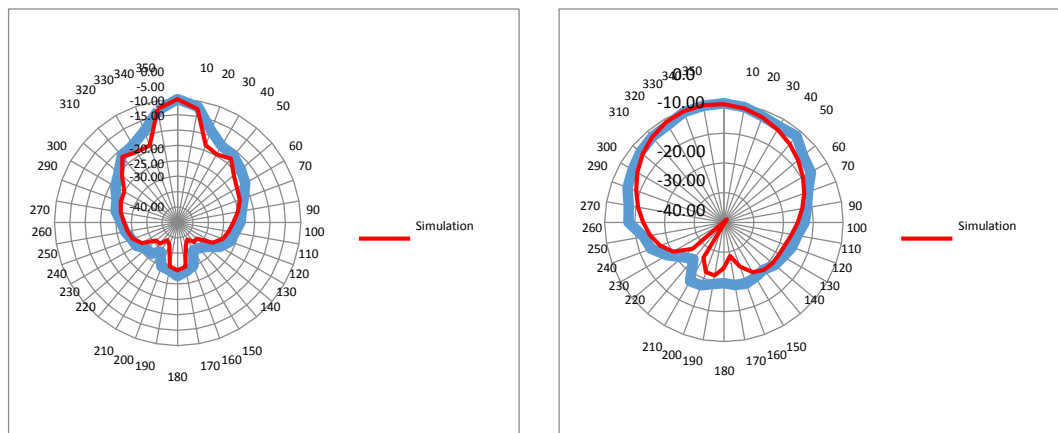
Gambar 4. 2 (a) Hasil pengukuran pola radiasi bidang Azimuth (b) Hasil pengukuran pola radiasi bidang elevasi
