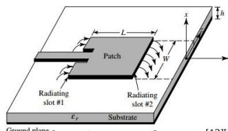
Gambar 2. 2 Struktur Antena Mikrostrip [13][14]
