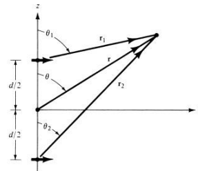
Gambar 2.4 Linier Array [3][20]
