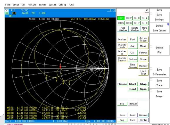
(b) Hasil Pengukuran Impedansi realisasi
