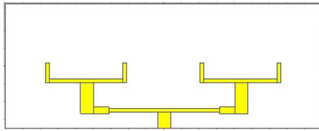
Gambar 3. 2 (a) Simulasi Antena susunan 4 elemen lapis 1
