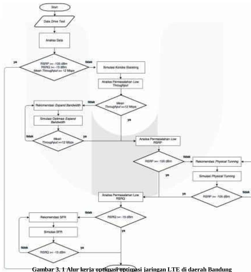
Gambar 3. 1 Alur kerja optimasi jaringan LTE di daerah Bandung
