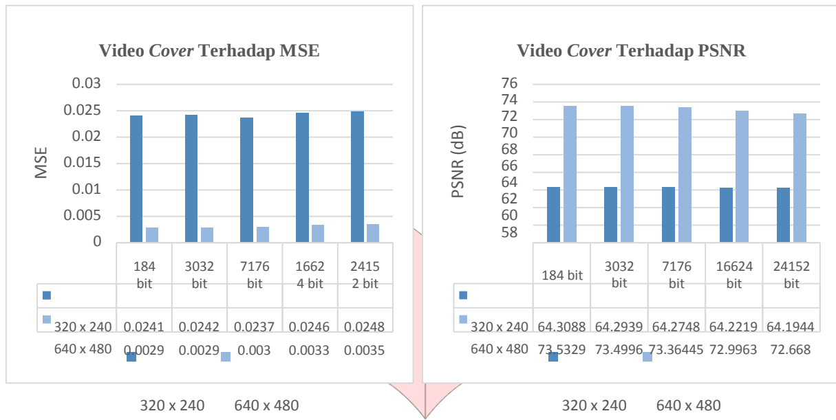
Gambar 3 (a) Pengaruh Panjang Pesan dan Ukuran Video Cover Terhadap MSE (b) Pengaruh Panjang Pesan dan Ukuran Video Cover Terhadap PSNR
