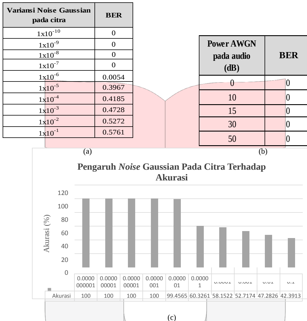
Gambar 4. (a) Pengaruh Noise Gaussian pada Citra Terhadap BER (b) Pengaruh Noise Gaussian pada Audio Terhadap BER (c) Pengaruh Noise Gaussian pada Citra Terhadap Akurasi
