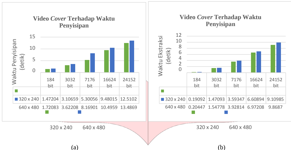
Gambar 2 (a) Pengaruh Panjang Pesan dan Ukuran Video Cover Terhadap Waktu Penyisipan (b) Pengaruh Panjang Pesan dan Ukuran Video Cover Terhadap Waktu Ekstraksi
