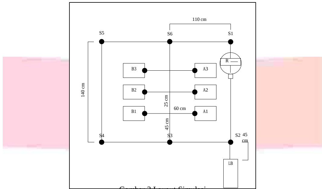
Gambar 3 Layout Simulasi
