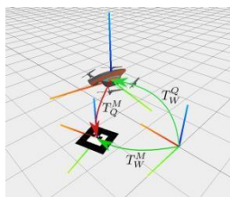
Fig. 3. Transformasi matriks pada quadcopter pendeteksi
