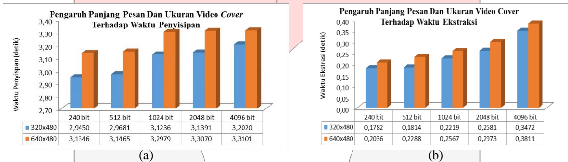
Gambar 3 (a) Pengaruh Panjang Pesan dan Ukuran Video Cover Terhadap Waktu Penyisipan (b) Pengaruh Panjang Pesan dan Ukuran Video Cover Terhadap Waktu Ekstraksi
