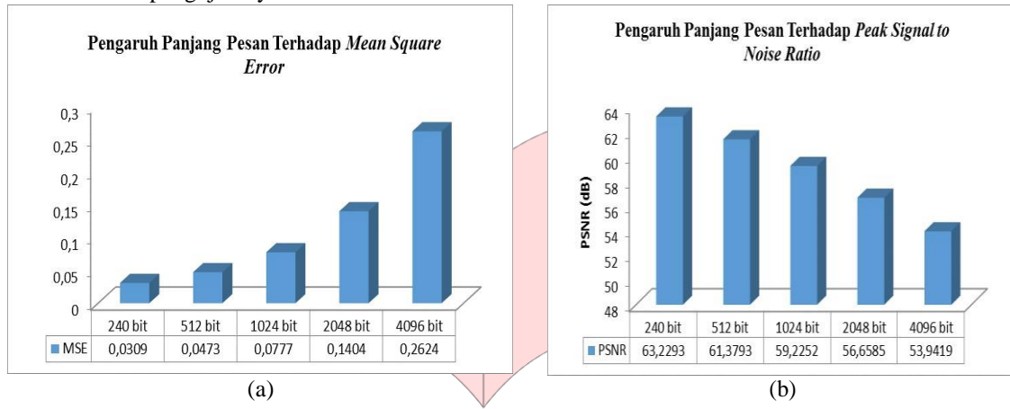
Gambar 4 (a) Pengaruh Panjang Pesan dan Ukuran Video Cover Terhadap MSE (b) Pengaruh Panjang Pesan dan Ukuran Video Cover Terhadap PSNR
