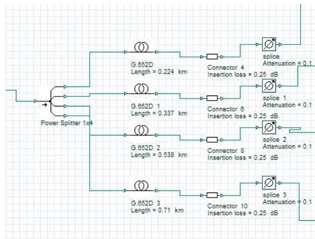
Gambar 5 Blok ODC
