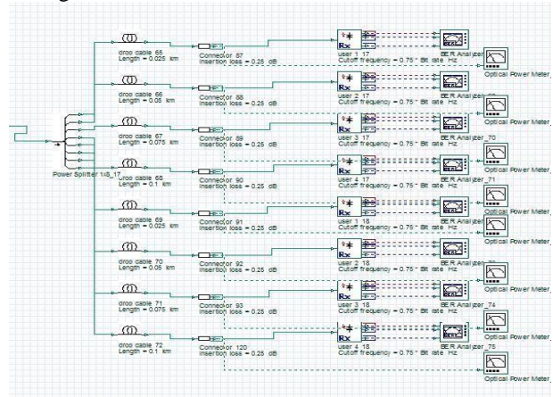
Gambar 6 Blok ODP ke Penerima
