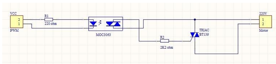
Gambar 3.3 Rangkaian Triac dan IC MOC
