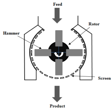
Gambar 2. Schematic Drawing Penggilingan Bahan di dalam Hammermill (Dabbour, 2015)
