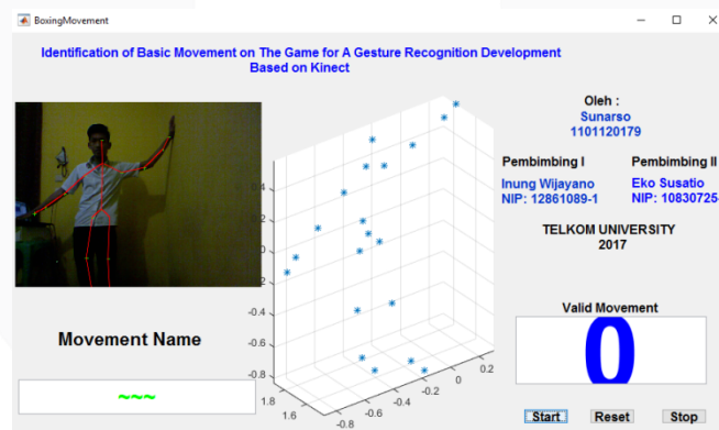
Gambar 4 Deteksi Pergerakan
