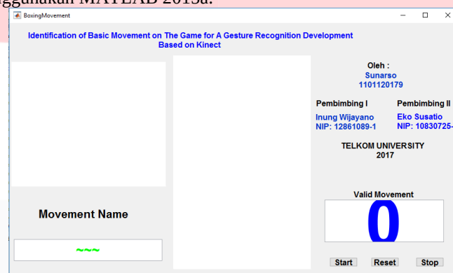
Gambar 6 GUI sistem
