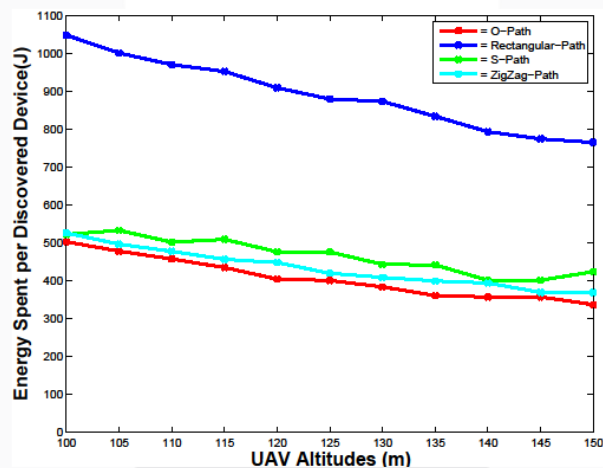
Gambar 4. 4 Energi yang dibutuhkan untuk mendeteksi satu perangkat
