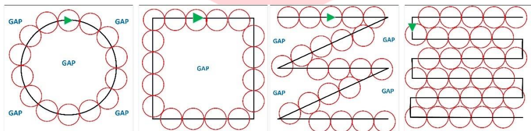
Gambar 3.2 Pola terbang UAV diadopsi dari [10]: (a) O-path (b) Rectangular-path
