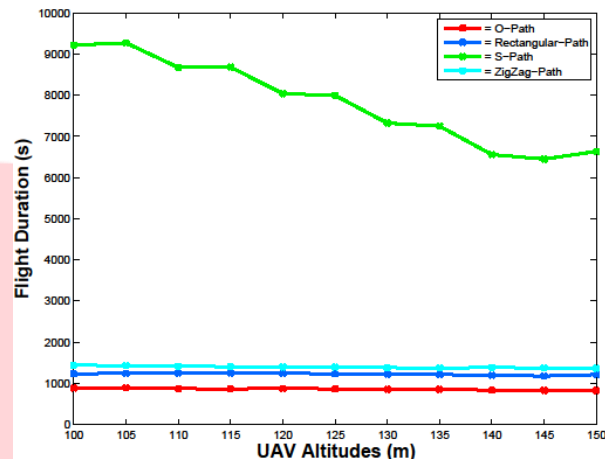
Gambar 4. 3 Durasi yang dibutuhkan
