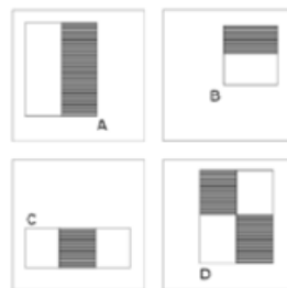
Gambar 2.3 Fitur haar
