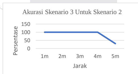
Gambar 3.4 Grafik akurasi skenario 3 untuk skenario 2
