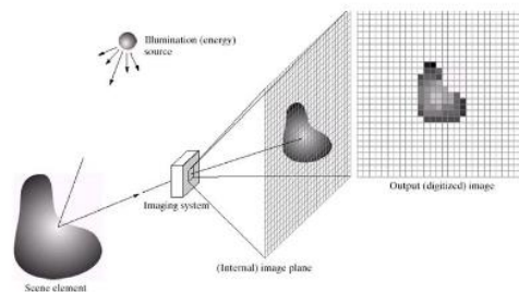
Gambar 2.1 Pemanfaatan sensor larik
