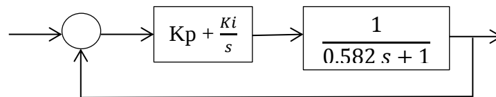
Gambar 5. Diagram blok close loop sumbu pitch dengan kendali PI
