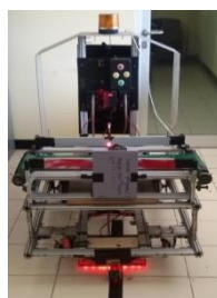
Gambar 3.2 Perancangan perangkat keras Coveyor Diverting System
