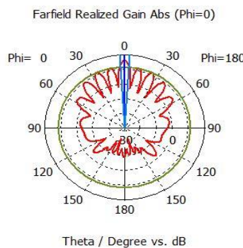
Gambar 12. Pola Radiasi Skenario 3 (2D)
