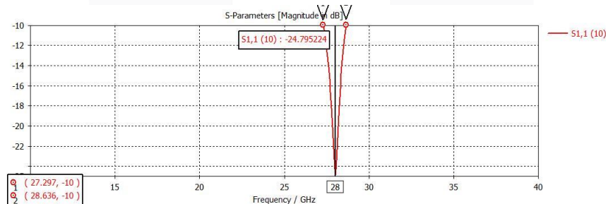
Gambar 15. Grafik S11 dari Antena menggunakan Konektor
