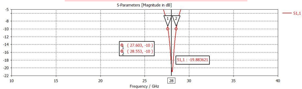
Gambar 5. Bandwidth dan S-Parameter antenna
