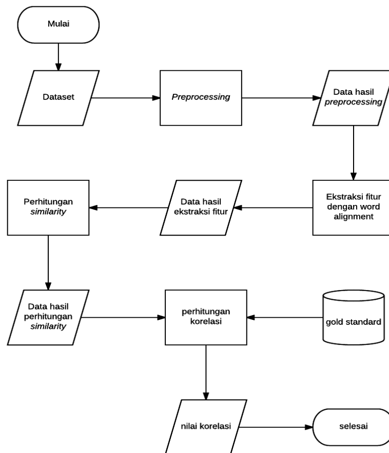
Gambar 3.1: Desain Sistem
