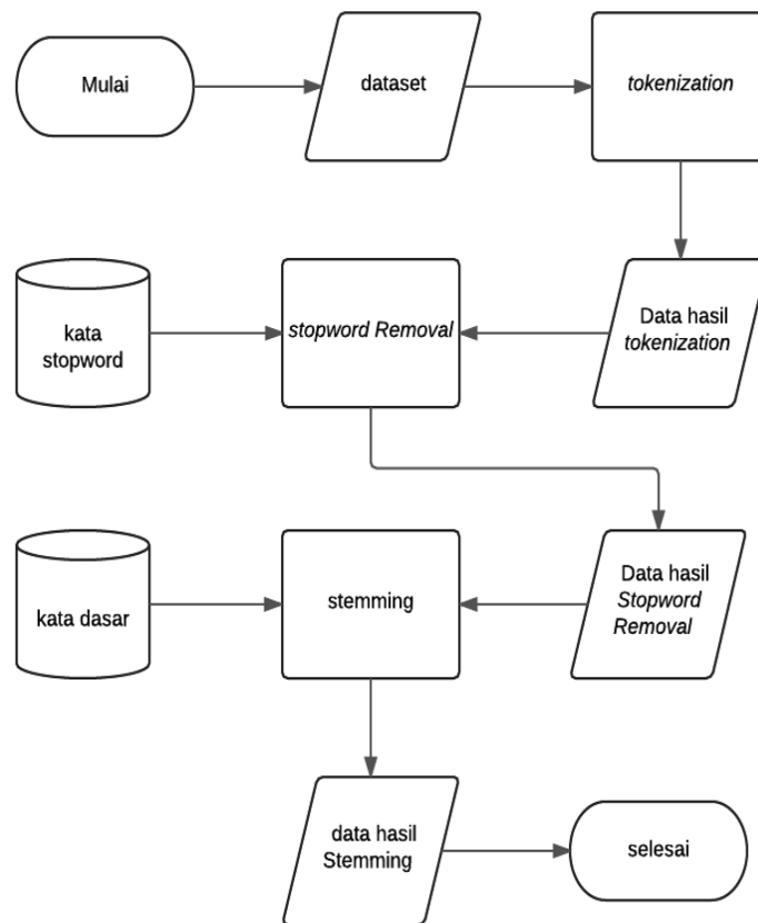
Gambar 3.2: Tahap Preprocessing
