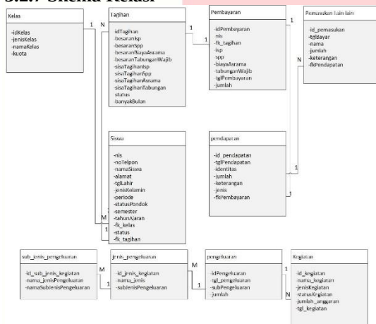
Gambar 3-7 Skema Relasi
