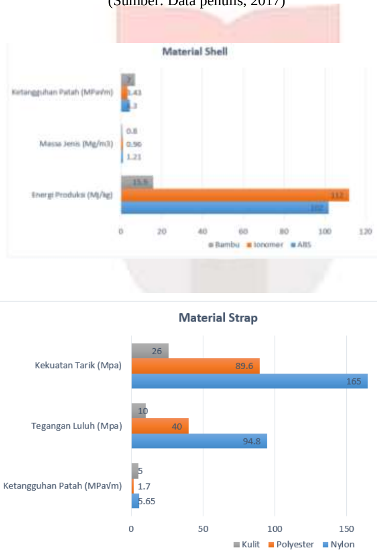
Gambar 1.2: Perbandingan Material tiap bagian
