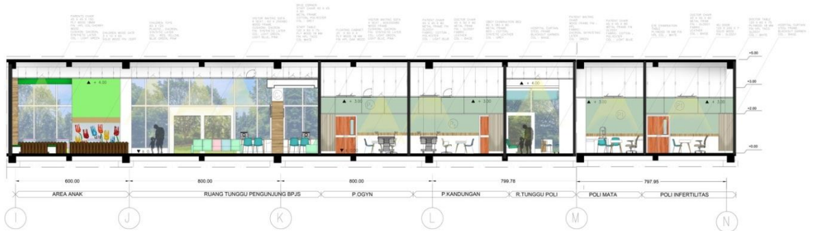
Gambar 3 Tampak C-C' Denah Khusus RSKIA Kota Bandung
