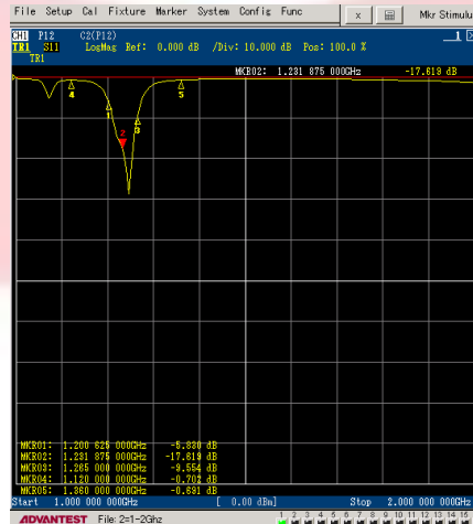
Gambar 7 Hasil Pengukuran Parameter S11 pada hasil realisasi
