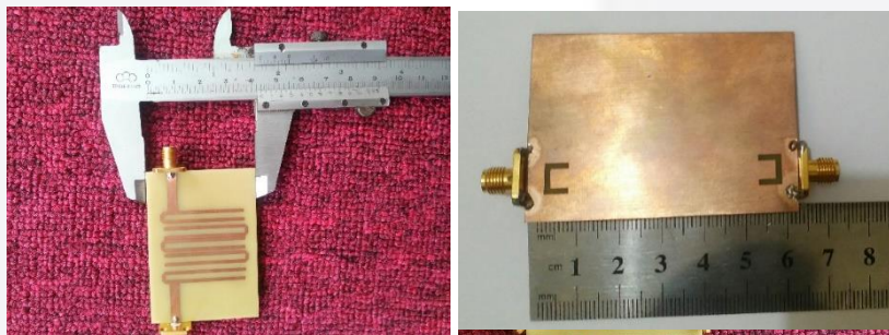
Gambar 5 Tampak Atas dan Bawah realisasi DGS Hairpin Line
