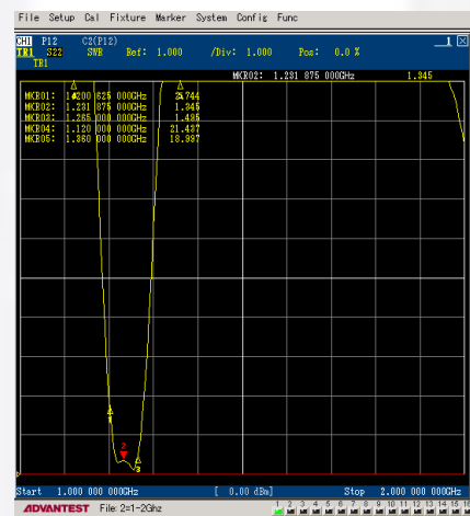
Gambar 8 Hasil pengukuran VSWR pada realisasi
