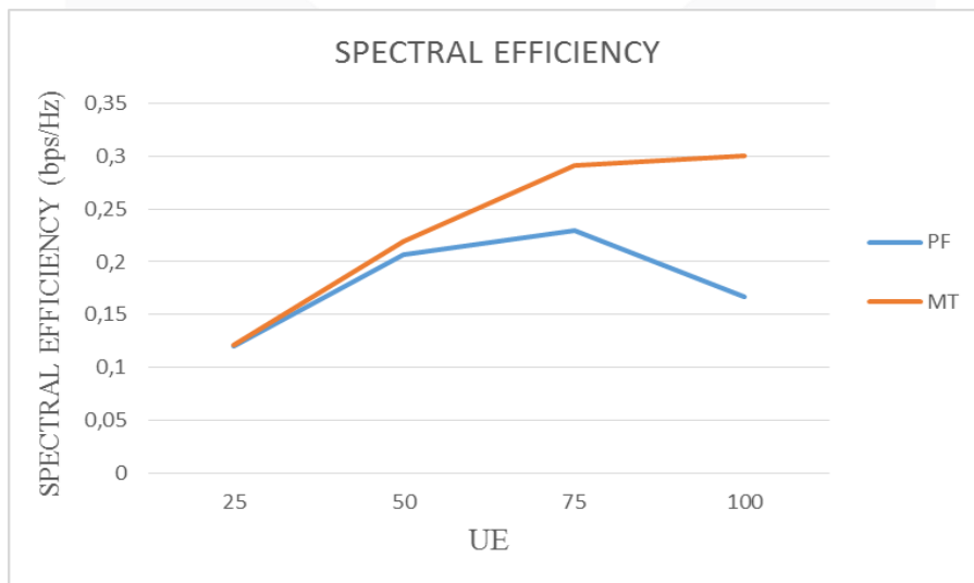
gambar 8 grafik perbandingan spectral efficiency PF dan MT
