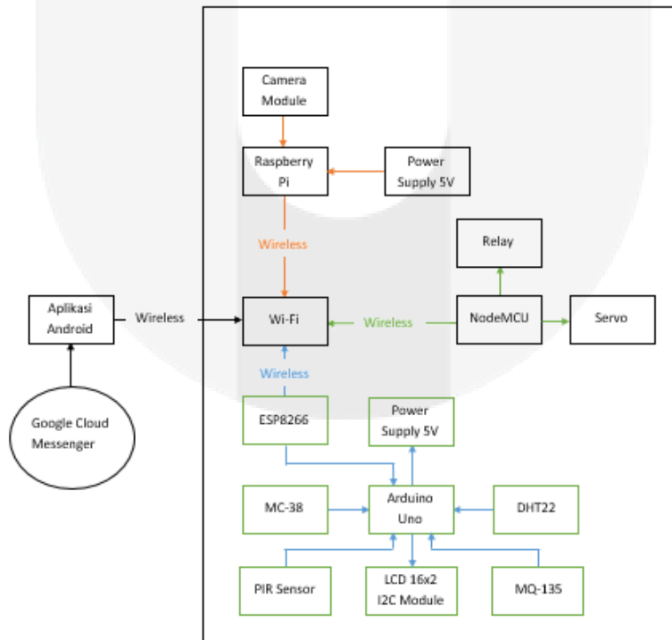
Gambar 2. Diagram blok sistem
