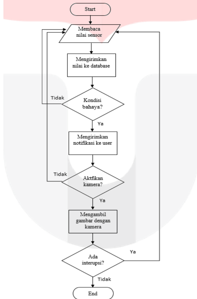
Gambar 3. Diagram alir sistem keamanan
