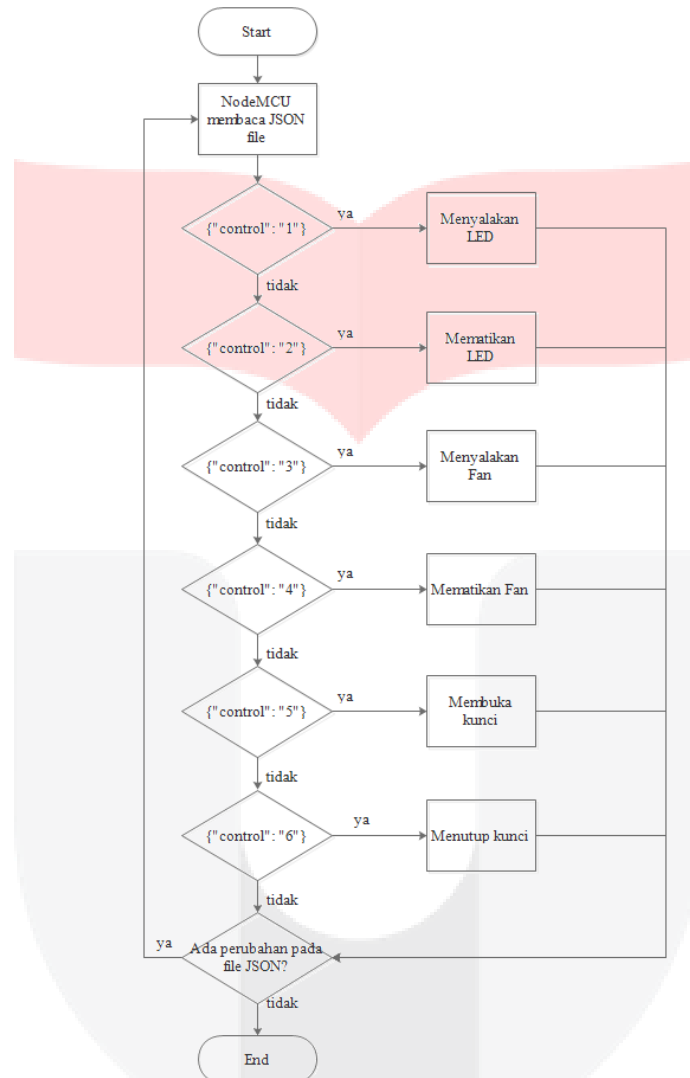
Gambar 4 Diagram alir sistem automasi
