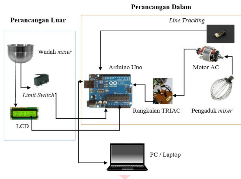
Gambar 3. Gambaran Perancangan Sistem Keseluruhan
