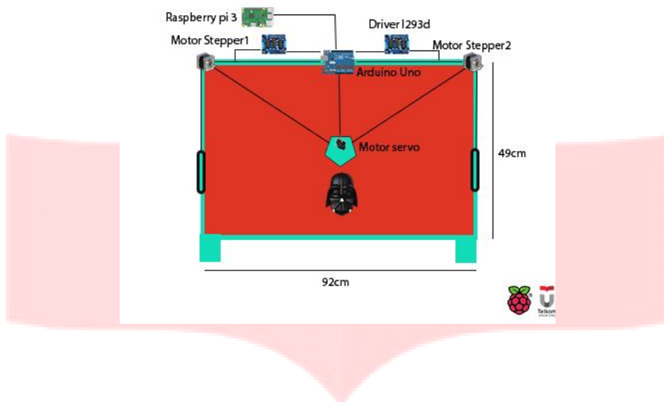
Gambar III – 1. Desain Plotter
