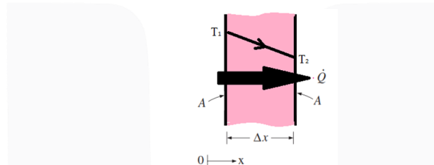
Gambar 1 Konduksi pada bidang datar ketebalan \Delta x dan luas A
