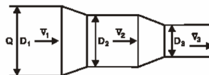
Gambar 2.1 Kontinuitas Aliran dalam Pipa
